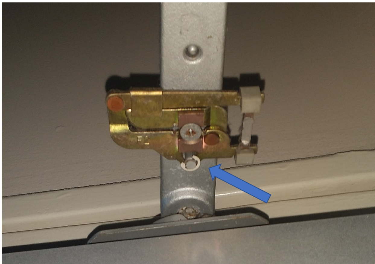
Eリング取り付け後（矢印がEリング）
